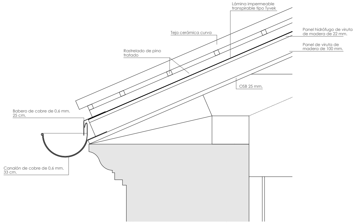
Detalle de alero escala 1/ 15
